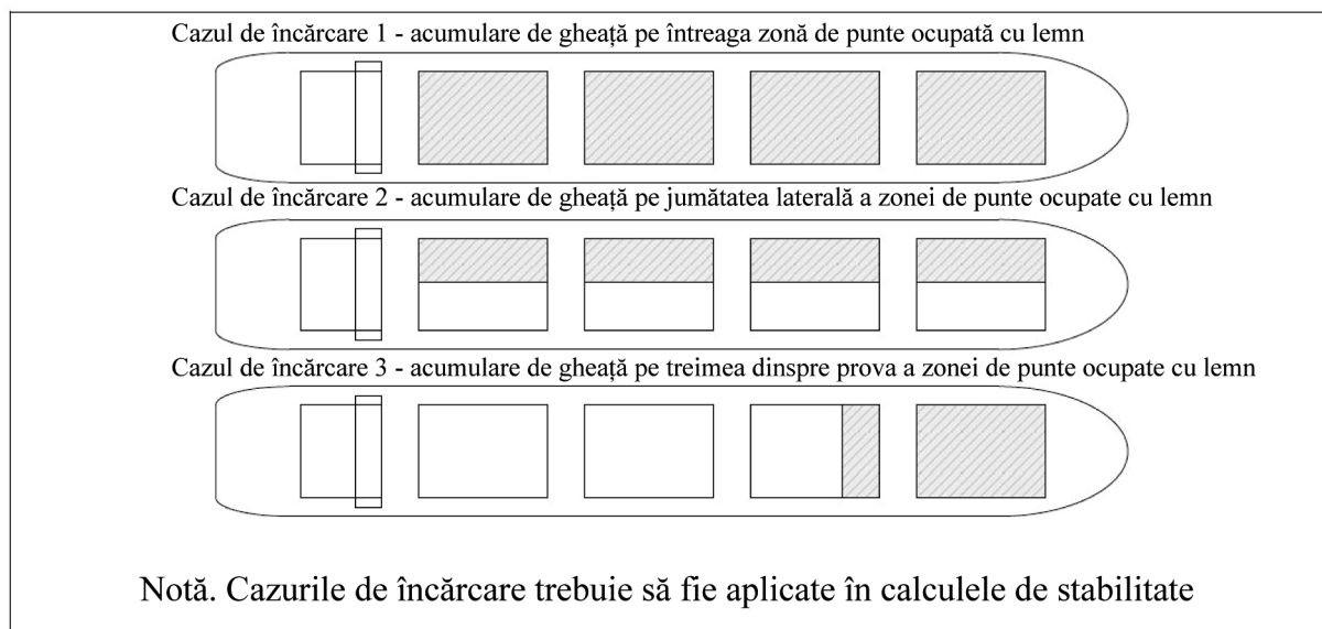
Figura 1 — Cazurile de încărcare ca urmare a acumulării de gheață pentru încărcătura de lemn pe punte
