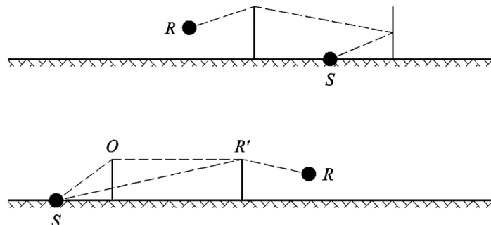
Figura 2.5.j: Diferența traiectoriei în prezența unei difracții: secțiunea transversală actuală (partea superioară), secțiunea transversală nedesfășurată (partea inferioară)
