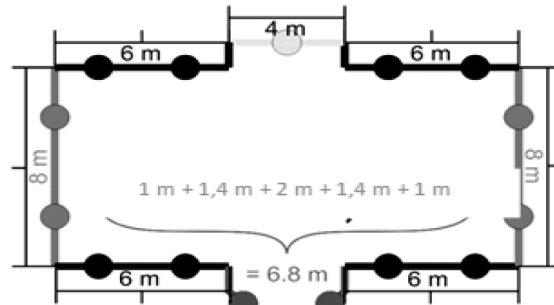
Figura a: exemplu de amplasare a receptoarelor în jurul unei clădiri conform procedurii pentru cazul 1.
