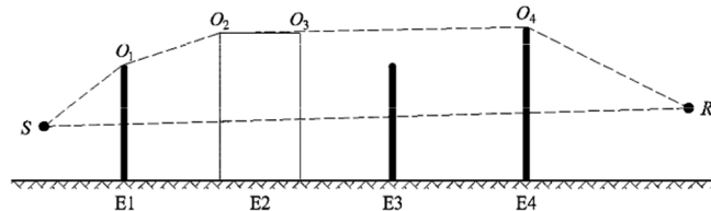
Figura 2.5.f: Exemplu de calcul al diferenței de cale în condiții favorabile, în cazul difracțiilor multiple În scenariul prezentat în figura 2.5.f diferența de cale este:
