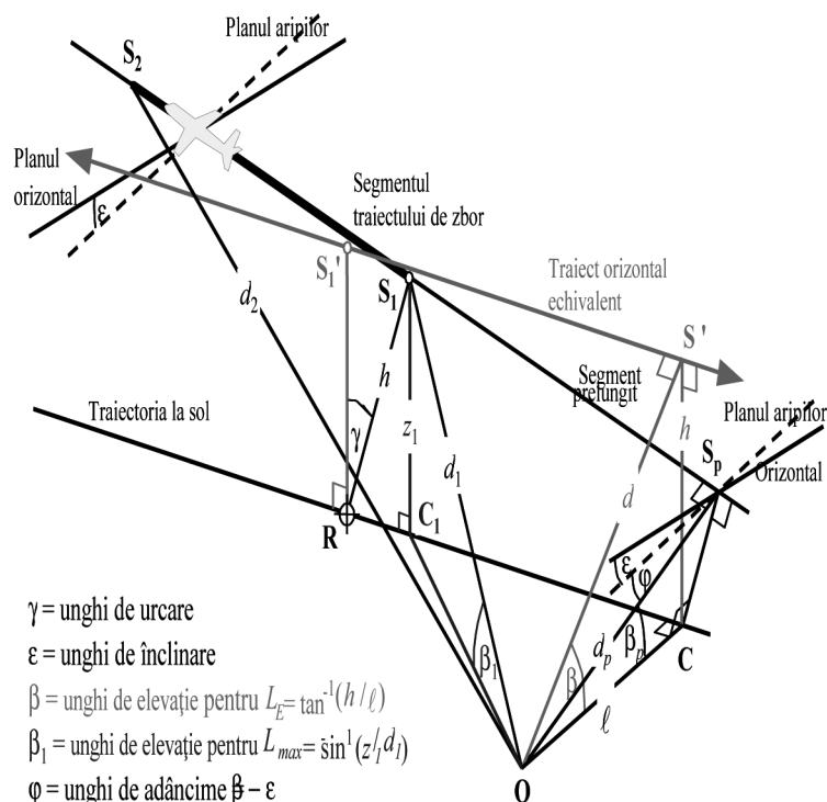
Figura 2.7.q: Observatorul în spatele segmentului
